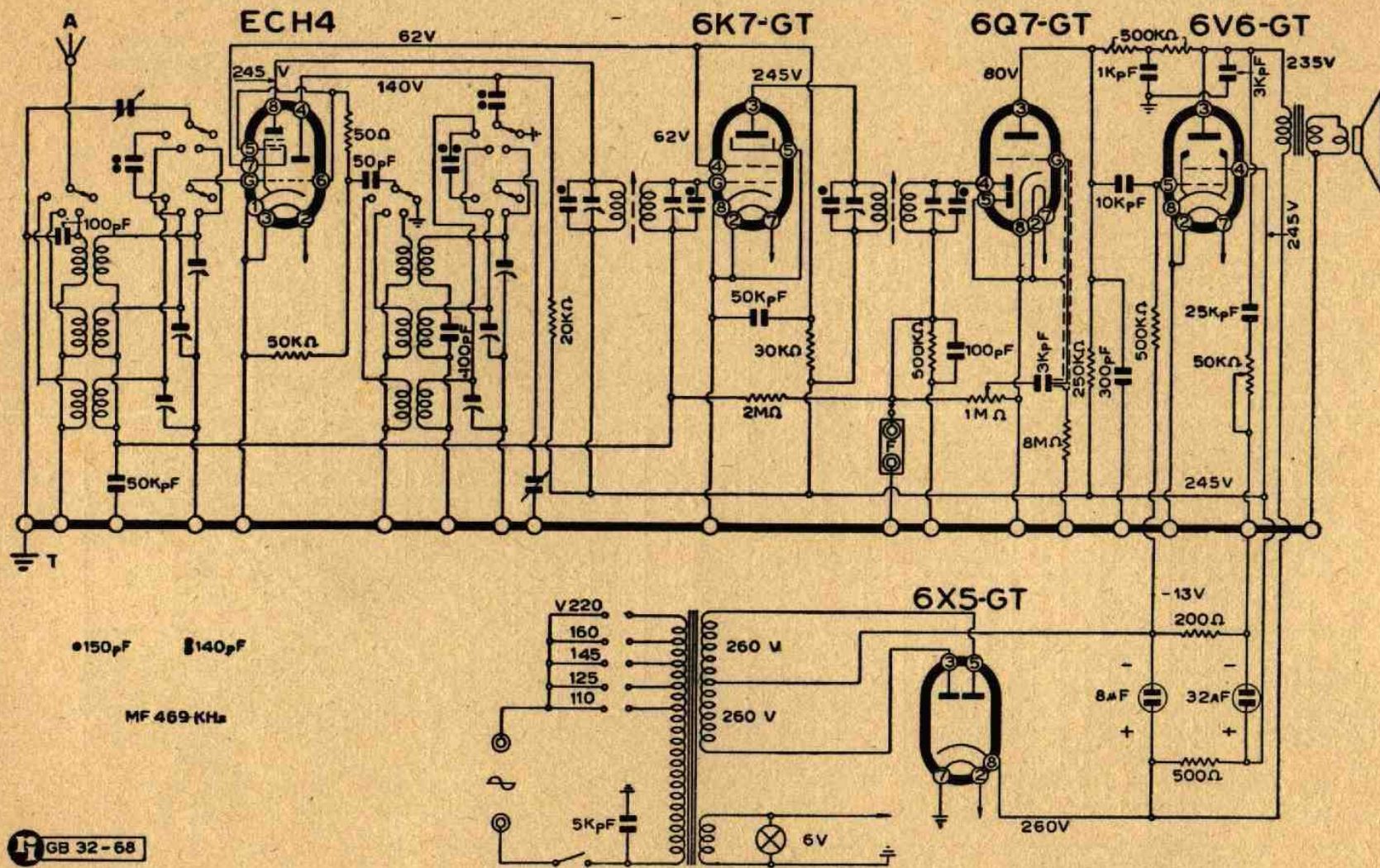
Lo schema elettrico del mod. S 530
